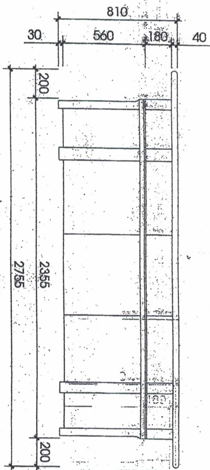
MẶT ĐUNG NGANG
