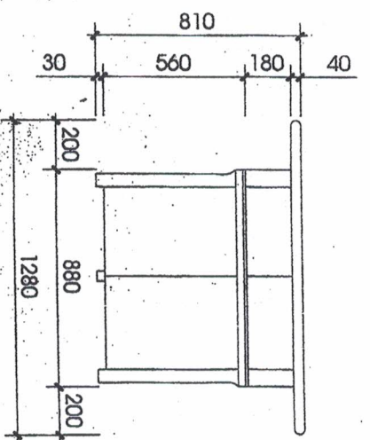
MẶT ĐỪNG DỌC
