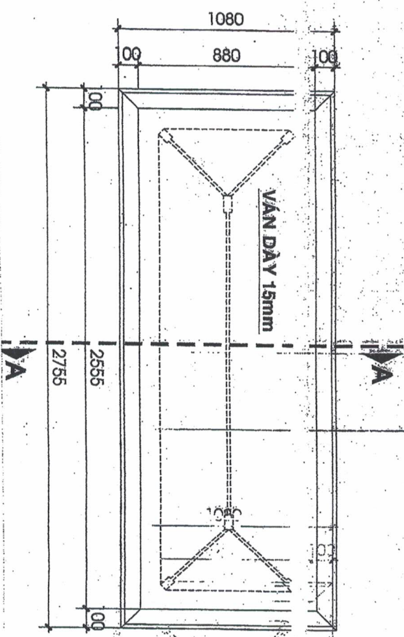
MẶT ĐUNG NGANG
