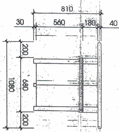
MẶT ĐUNG DỌC
